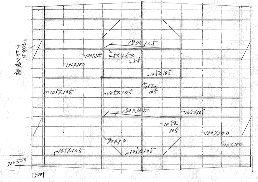
小屋伏図 S=1/100
