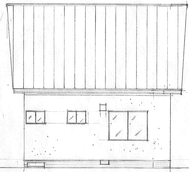
立面圖 右側面 S=1/100
