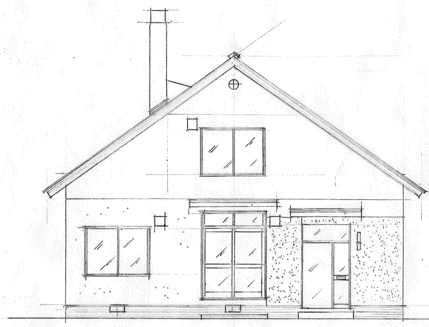
立面圖 正面 S=1/100
