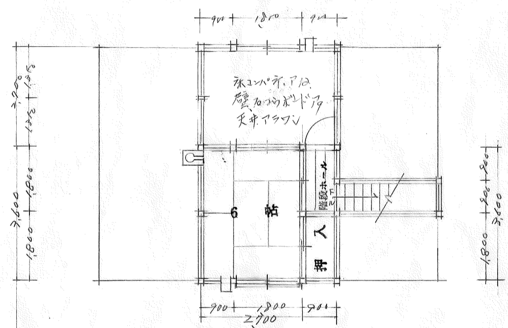
2階平面圖 S=1/100 床面積 15.39 M 2
