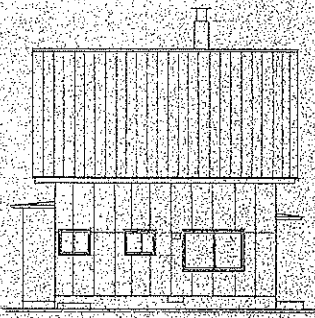
立面图左侧面 1/60
