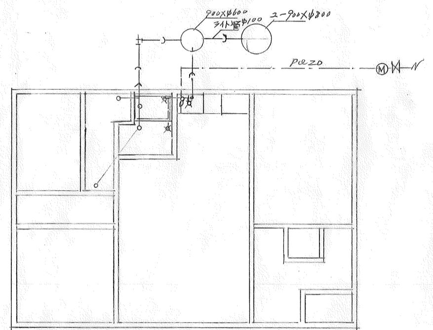
給排水設備 S=1/100
