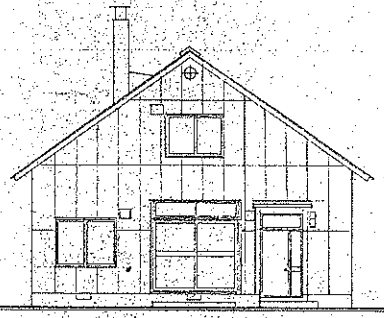
立面图正面 1/60
