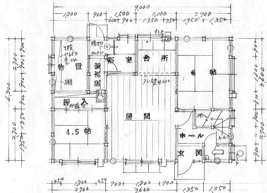
1階平面圖 S=1/100 建築面積 56.7 M 2 床面積 56.7 " 延面積 72.07 "
