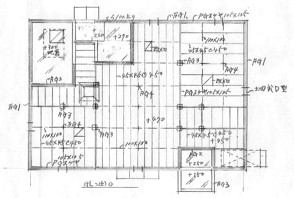
基礎伏図床組図 S=1/100
