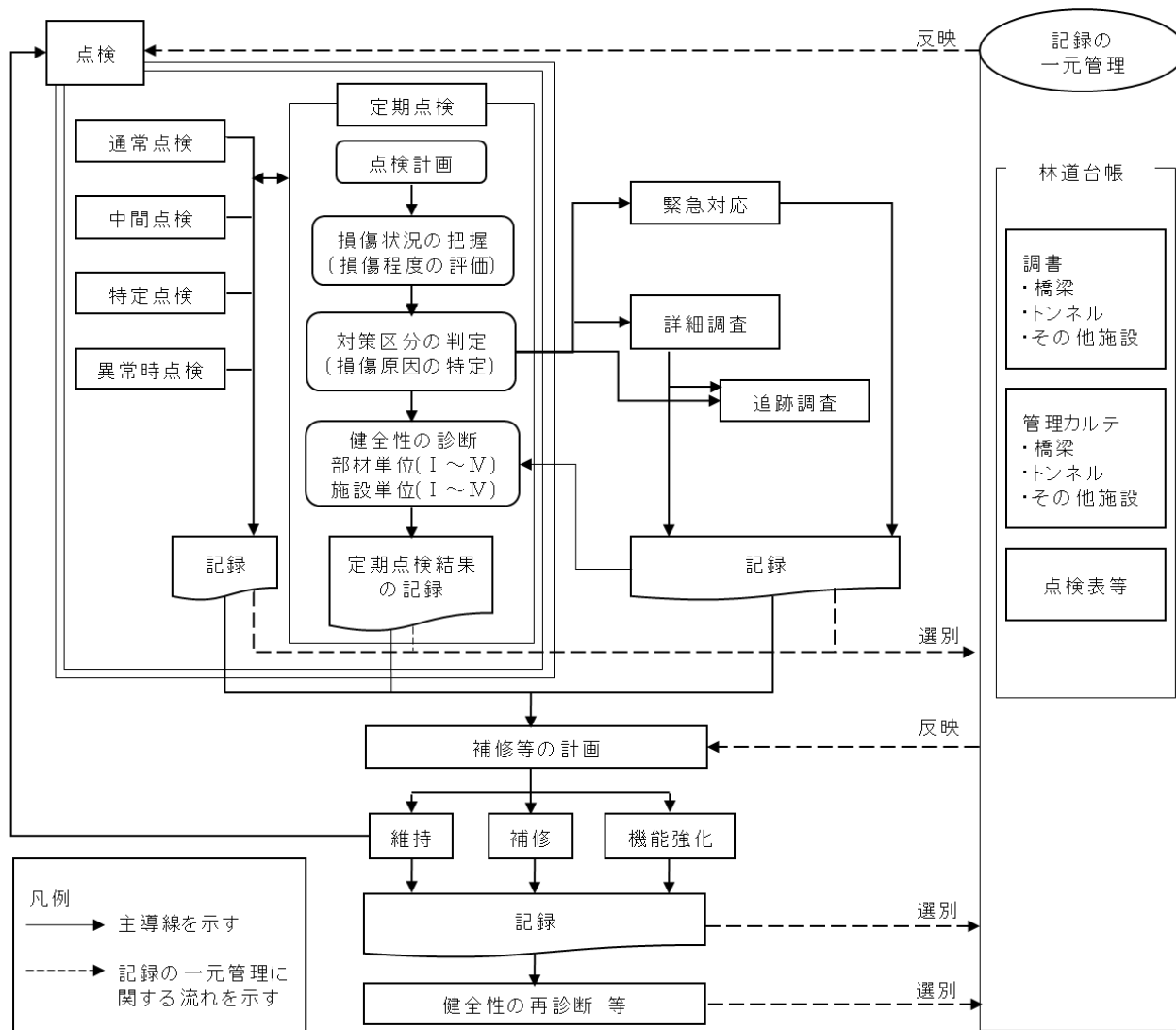
図1 定期点検と健全性評価のフロー
