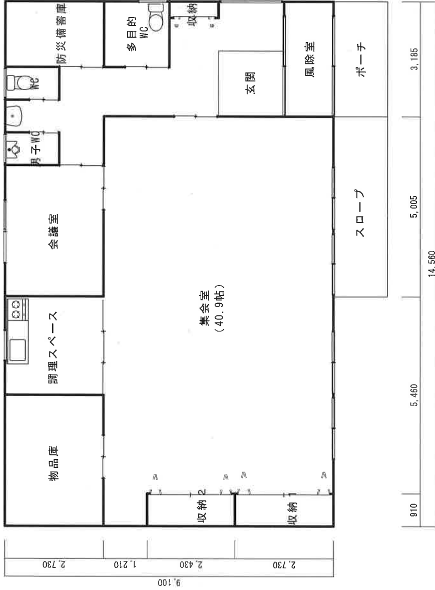
平面図 S:1/100
