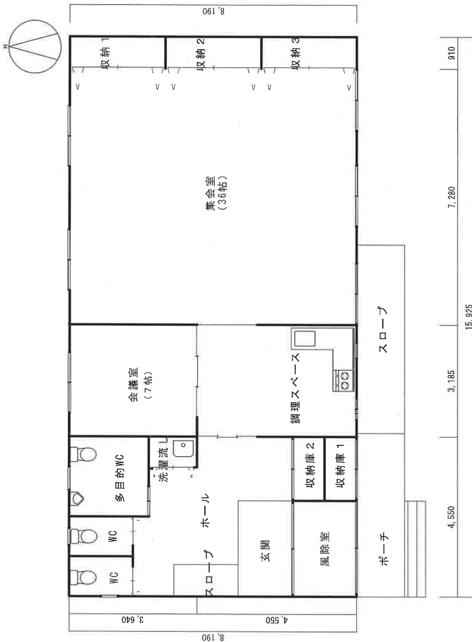
平面図 S=1/100
