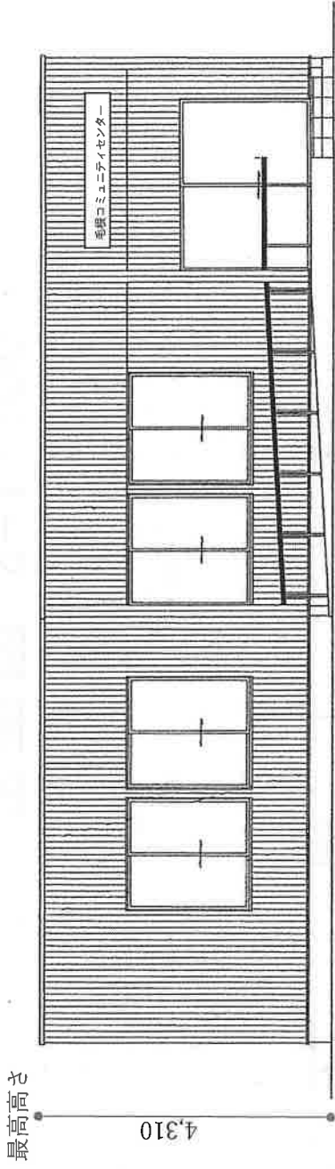
南立面図
