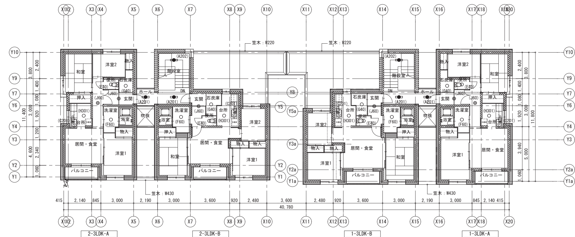
2階平面図
