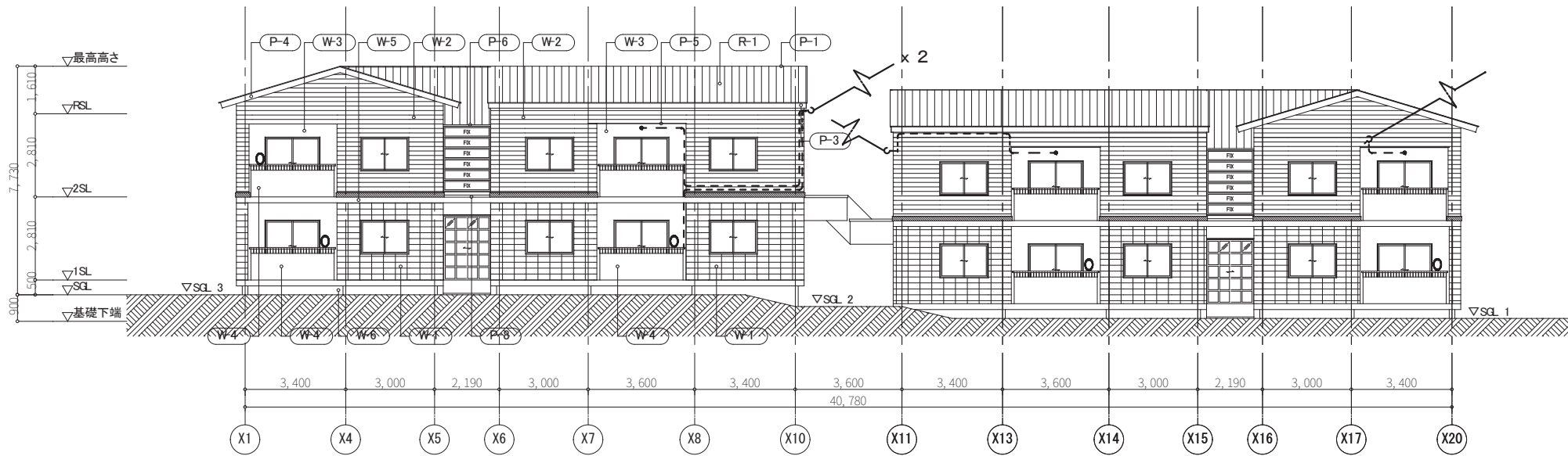
南側立面図
