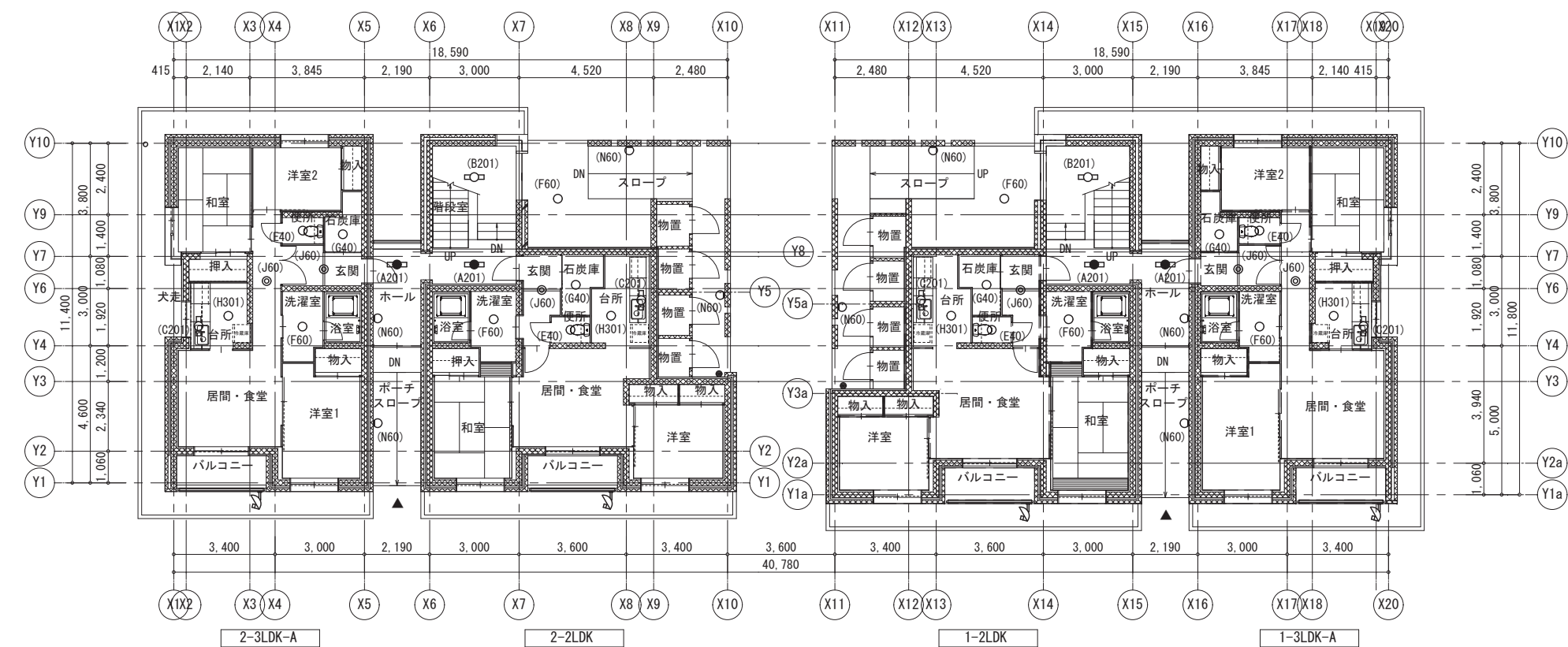
1階平面図
