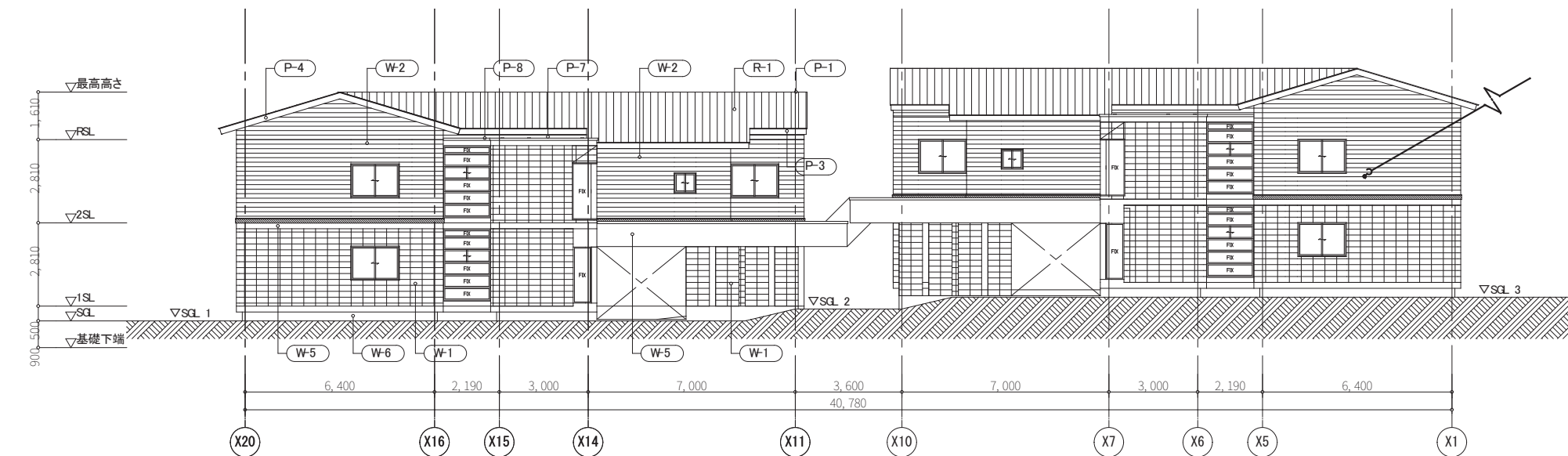
北側立面図
