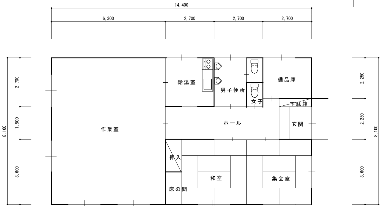
平面図（既存）
