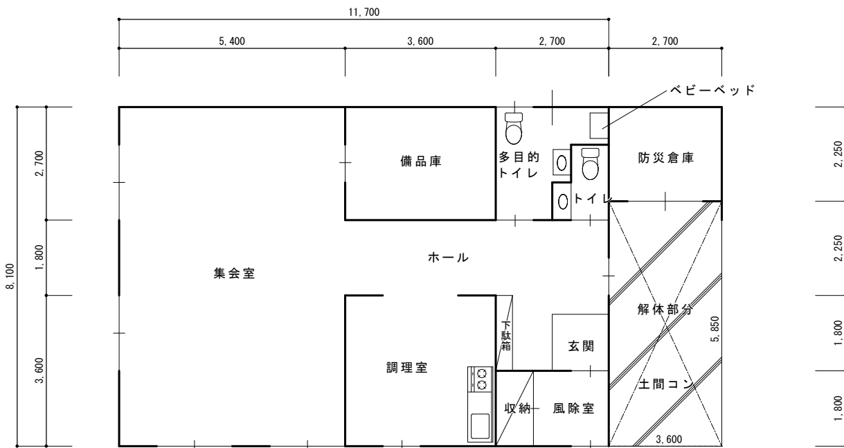
平面図（改修案）※実施設計により変更になることもあります。
